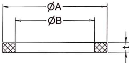
Section D-D
