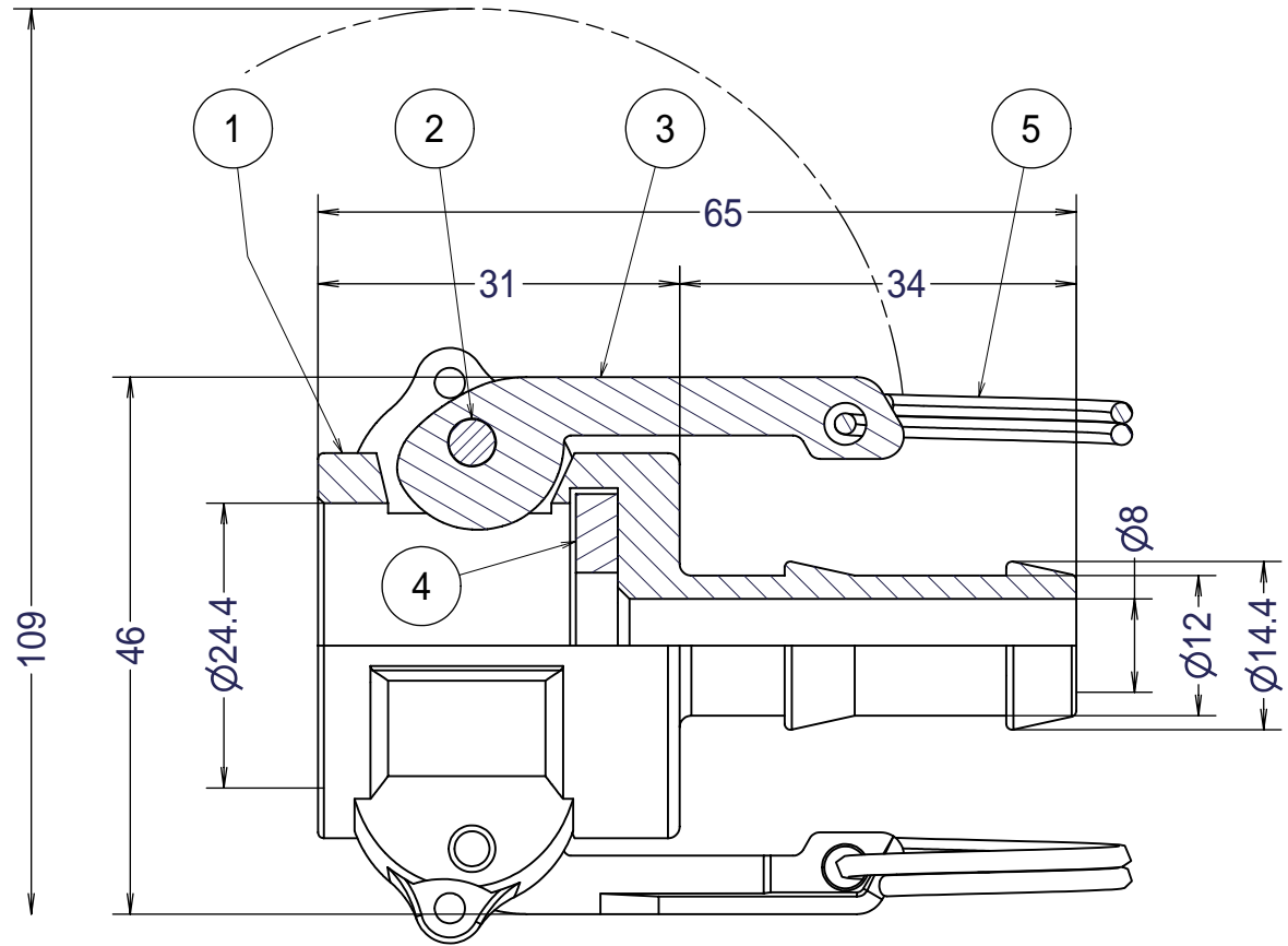
Section D-D
