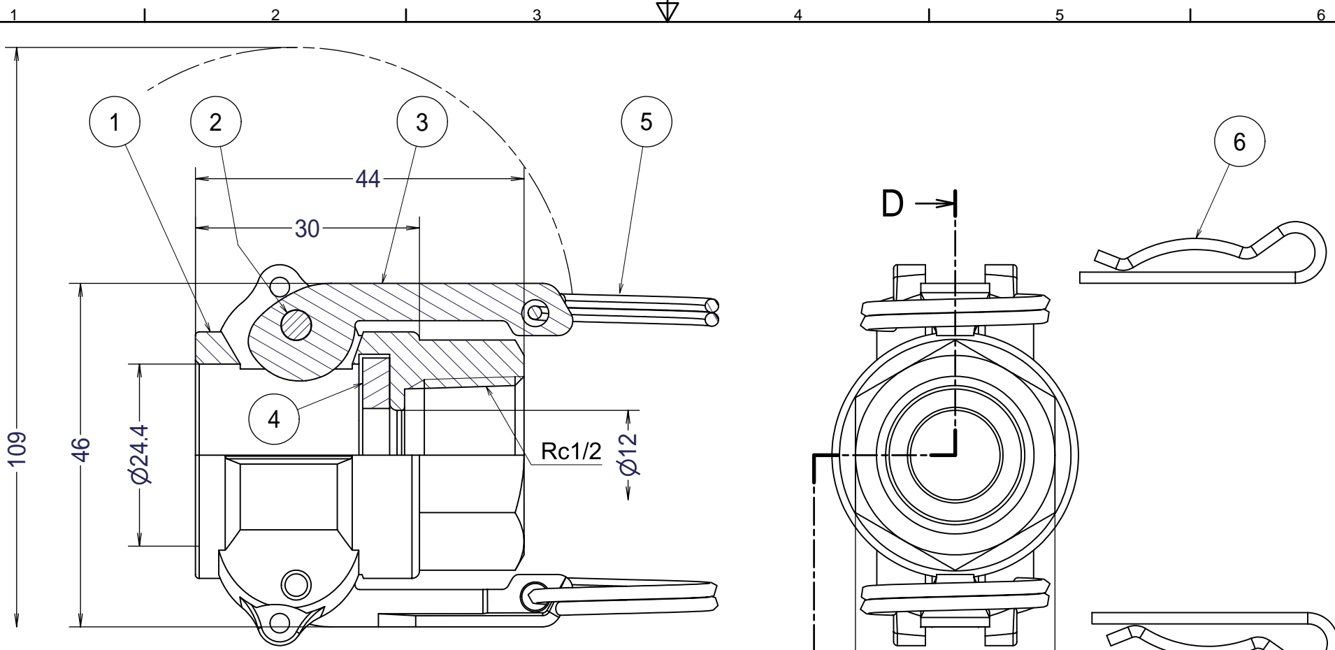
Section D-D
