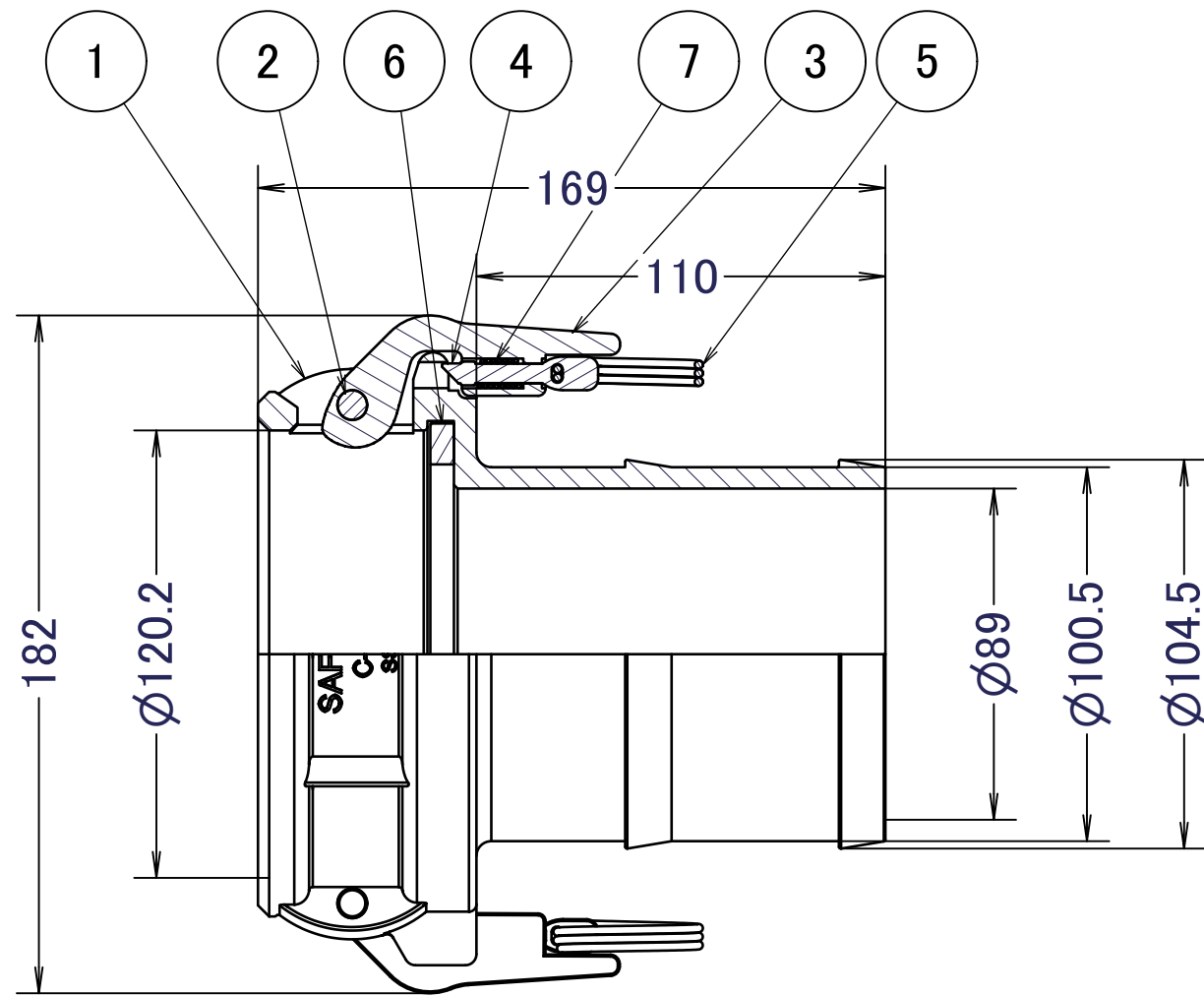
Section D-D
